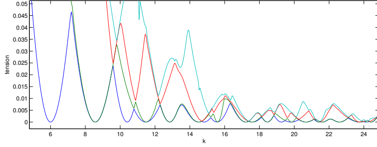
FIGURE 3.7 – Tension pour une plaque carrée encastrée
