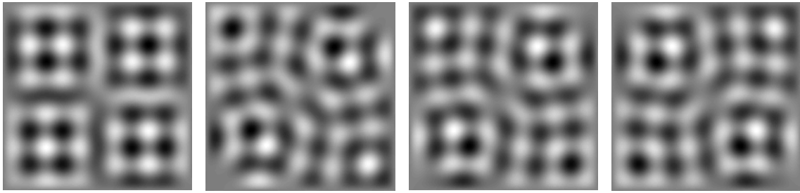
FIGURE 3.5 – Base de l'espace propre pour k = \sqrt{125}\pi . La dimension de l'espace d'approximation est de 73.
