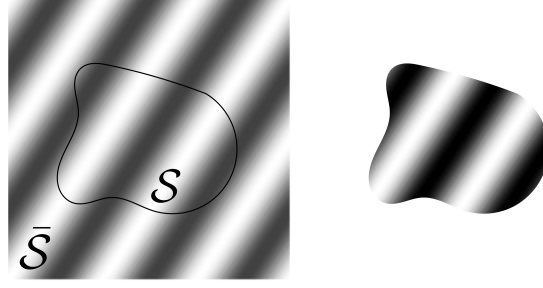
FIGURE 6.2 – Construction des atomes du dictionnaire. À gauche, le domaine \bar{\mathcal{S}} sur lequel est construit les vecteurs de base de la transformée de Fourier, et la forme de la plaque \mathcal{S} . À droite, un atome du dictionnaire.
