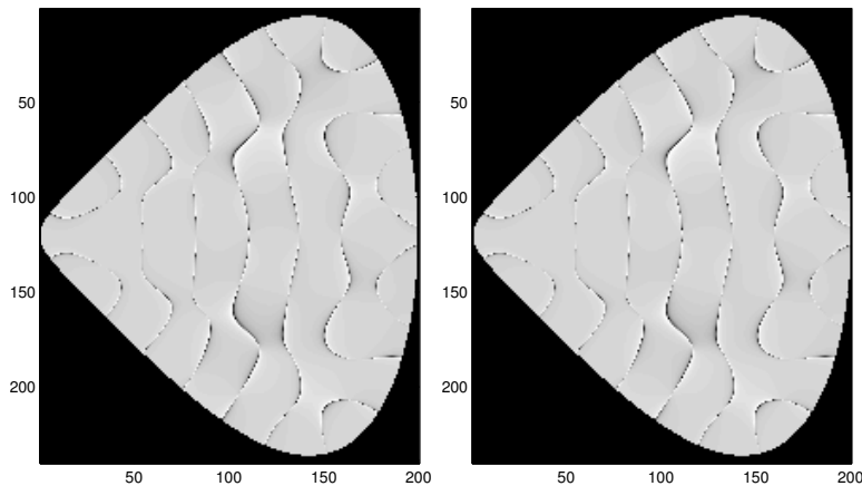
FIGURE 8.2 – Corrélations du dictionnaire réverbéré avec les mesures pour deux source différentes, à une fréquence proche d'une fréquence propre
