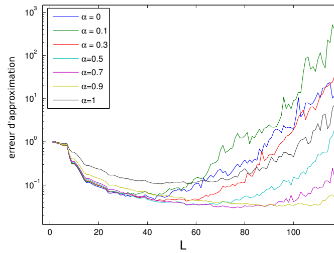
FIGURE 4.1 – Erreur de reconstruction en fonction de L , pour 400 mesures et différentes proportions \alpha d'échantillons sur le bord
