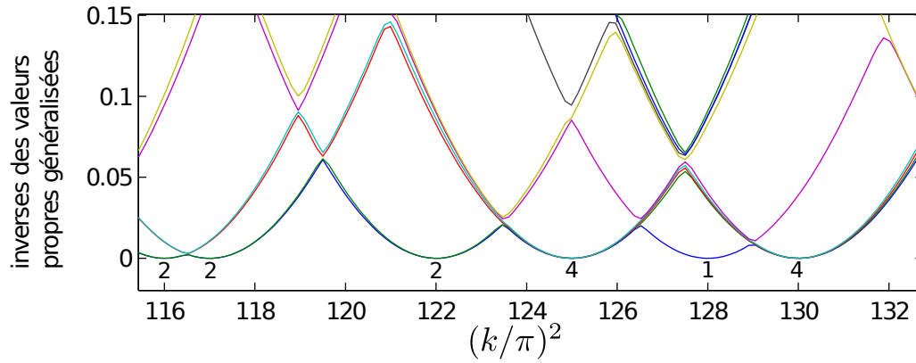
FIGURE 3.4 – Agrandissement de la figure précédente. Les ordres des fréquences propres sont indiqués. Ce sont le nombre de valeurs propres généralisées de 3.8 atteignant 0.
