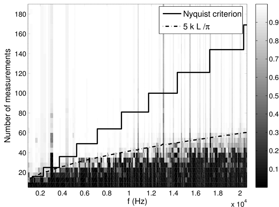
FIGURE 7.14 – Qualité de la reconstruction (mesurée par la corrélation) du mode en fonction de sa fréquence et du nombre d'échantillons utilisés. La limite du theoreme d'échantillonnage est indiquée en trait gras.
