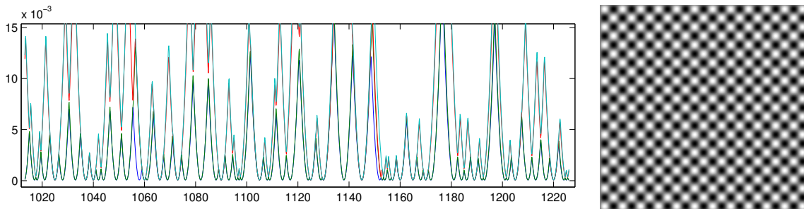
FIGURE 3.6 – Inverses des valeurs propres de 3.8 pour le même intervalle que la figure 3.2. Le mode (simple) à k = \sqrt{1058}\pi est donné. La dimension de l'espace d'approximation est de 172, alors que le calcul par éléments finis nécessiterait plus de 10 000 éléments.
