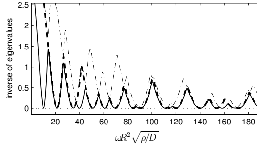
FIGURE 3.10 – Tension pour la plaque circulaire encastree.
