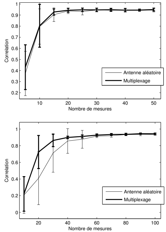
FIGURE 4 – Corrélations moyennes et écarts-types, pour les modes à 402 Hz (gauche) et 2180 Hz (droite), pour 30 réalisations d'antenne aléatoire et de multiplexage gaussien complet.
